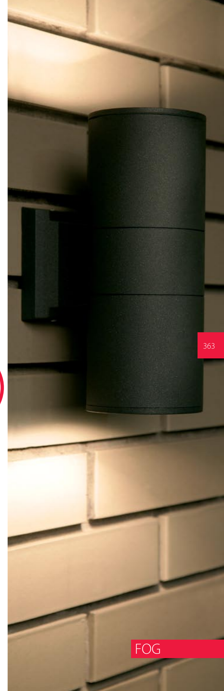
3402 FOG I kinkiet ↓ 20 cm → 17 cm 1 x E27 max 60W IP 44
