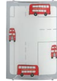
2957 BUS 1 ↓ 22 cm ↔ 15 cm 1 x E14 max 60W
