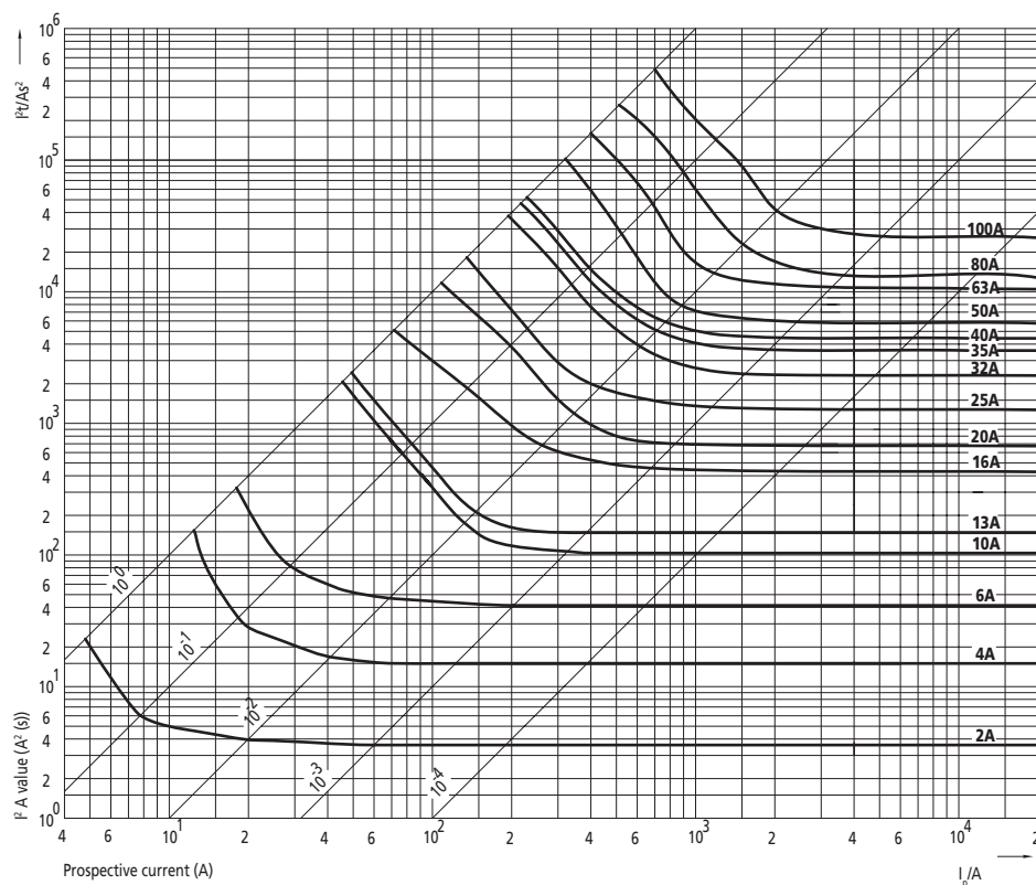
Tavná charakteristika I^2 t / A, \text{ gG/gL}
