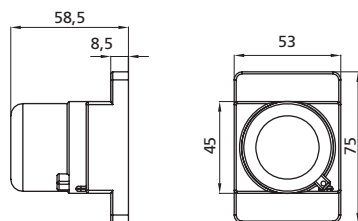
Ochranný kryt pre poistkové spodky EZN 25 a EZV 25
