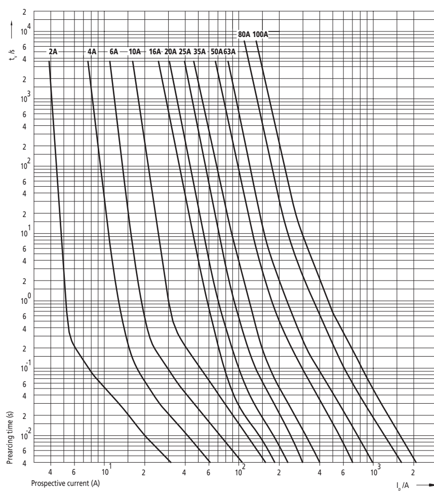
Časová charakteristika I/t \text{ DZ}
