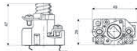
Poistkový spodok DI
