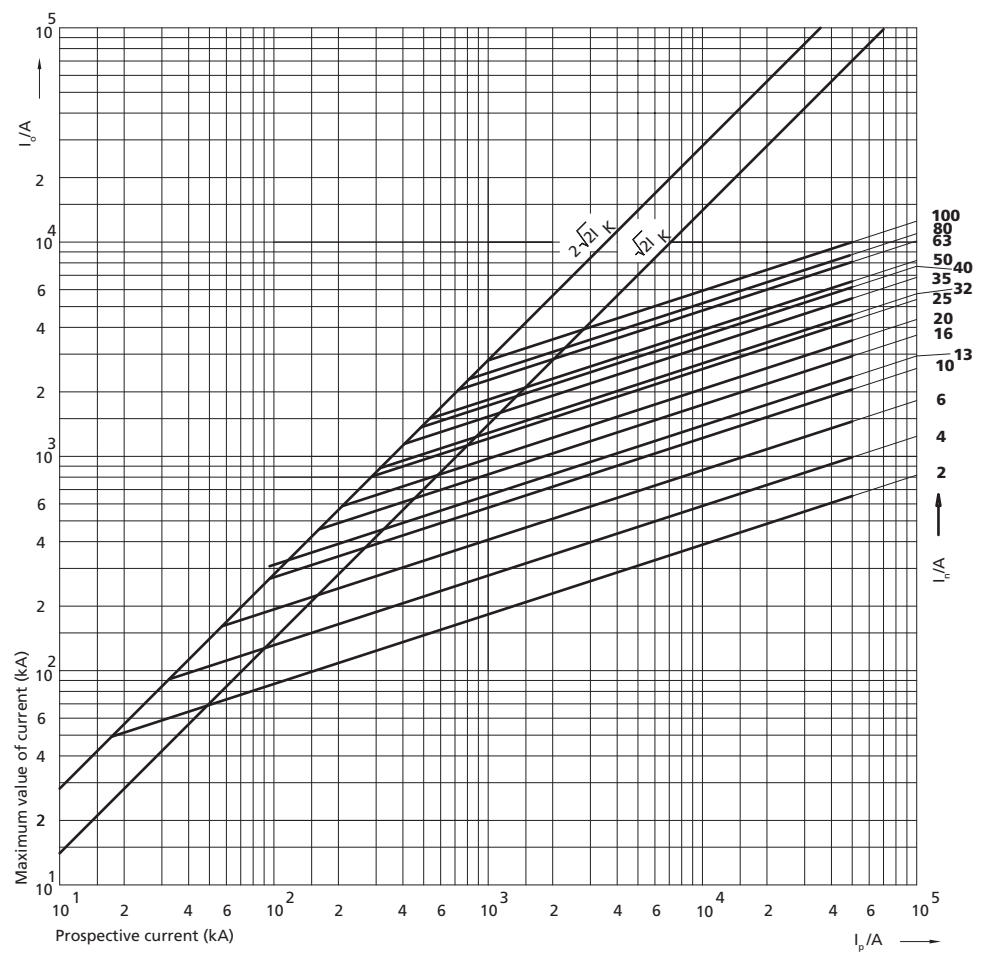
Skratová charakteristika I^2t
