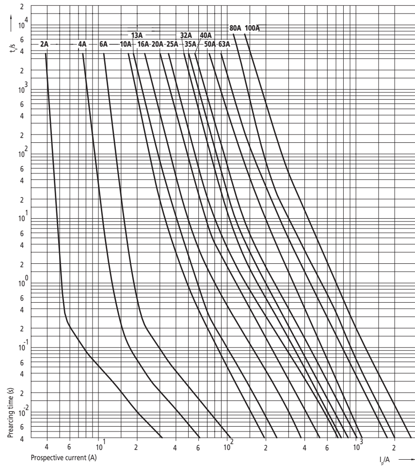
Časová charakteristika I/t, gG/gL
