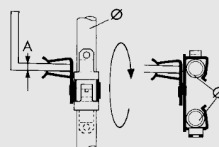
H-MAC2 PŘÍCHYTKA
