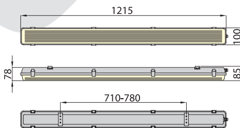
wymiary oprawy
