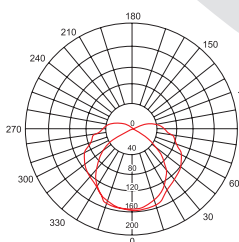
wykres rozsyłu światła
