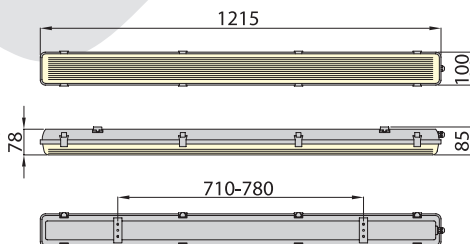
wymiary oprawy
