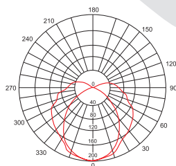
wykres rozsyłu światła
