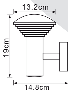
wymiary oprawy
