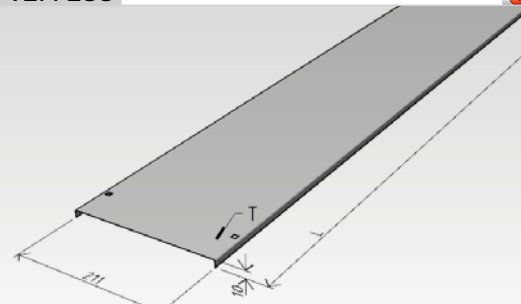
víko žlabu VZM 200
