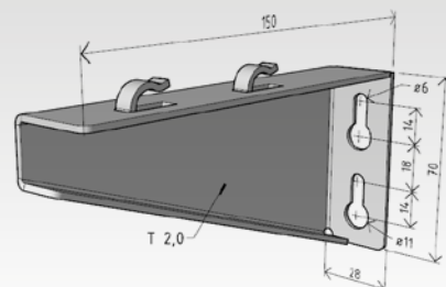
nosník NNM 150
