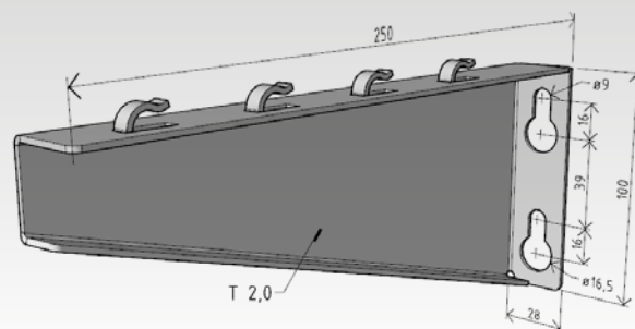
nosník NNM 250
