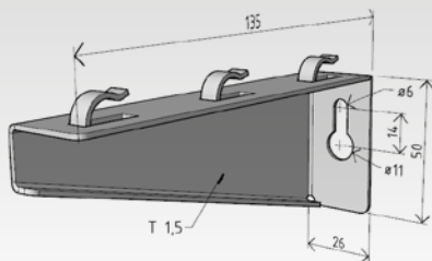
nosník NNM 100
