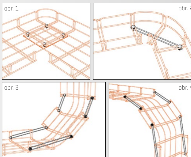
ukázka montáže
