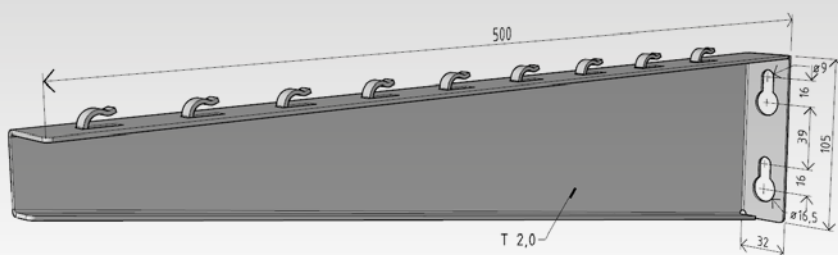
nosník NNM 500
