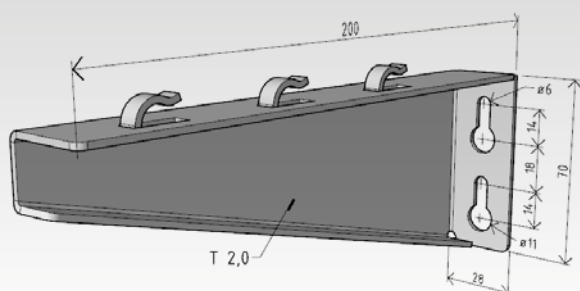
nosník NNM 200
