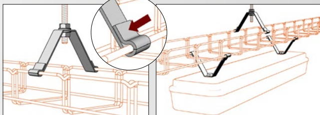
ukázka montáže
