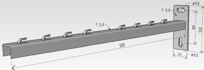
nosník NPZM 500
