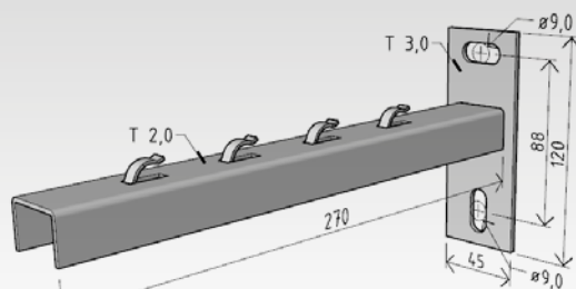
nosník NPZM 250
