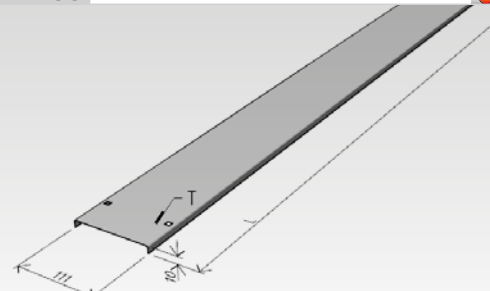
víko žlabu VZM 100
