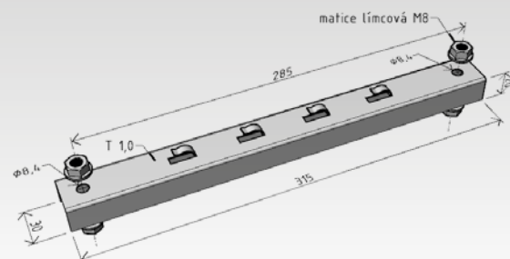
podpěra PZM 250
