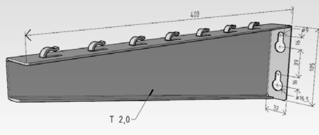
nosník NNM 400
