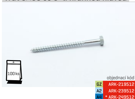
vrut 6×80 se 6-ti hrannou hlavou
