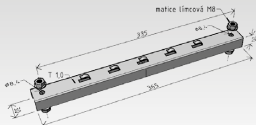
podpěra PZM 300
