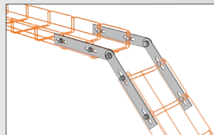
ukázka montáže
