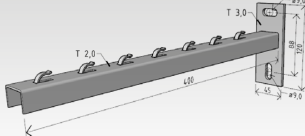
nosník NPZM 400
