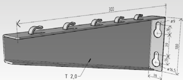
nosník NNM 300
