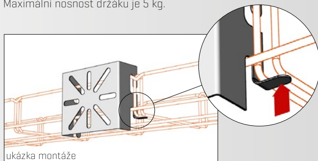
ukázka montáže
