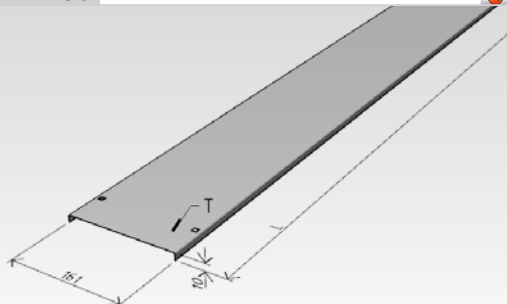
víko žlabu VZM 150
